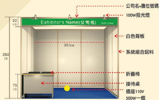
《3MX3M基本攤位裝潢設備圖》
